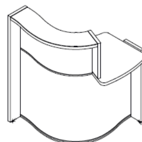
Module autonome, H110/74 cm Accueil bas à Droite ou à Gauche
